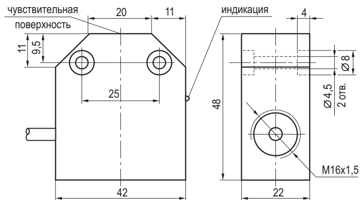
Габаритный чертеж
