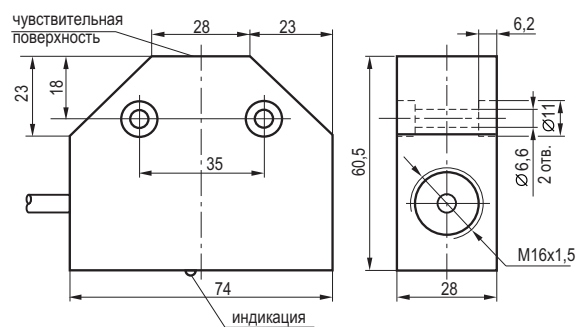
Габаритный чертеж
