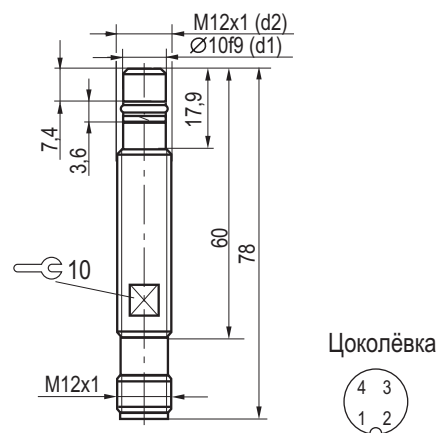
Схема монтажа
