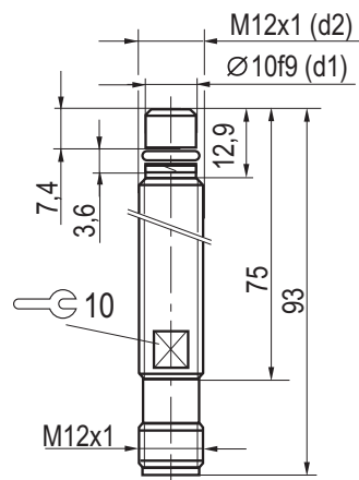
Габаритный чертёж
