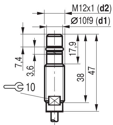
Габаритный чертеж
