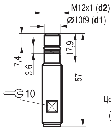
Габаритный чертеж
