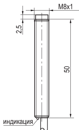
Габаритный чертеж
