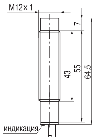
Габаритный чертеж
