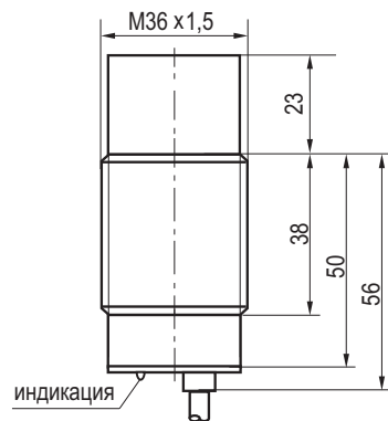
Габаритный чертеж
