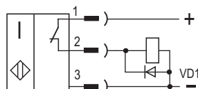
Схема подключения индуктивной нагрузки
