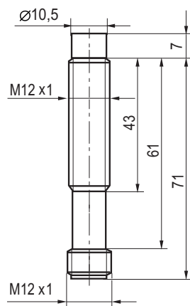
Габаритный чертеж
