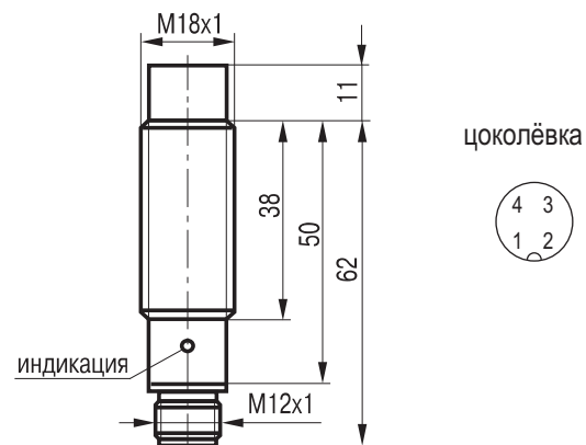
Габаритный чертеж
