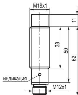
Габаритный чертеж
