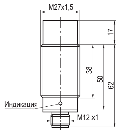
Габаритный чертеж
