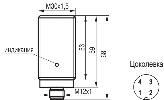
Габаритный чертеж
