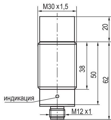
Габаритный чертеж
