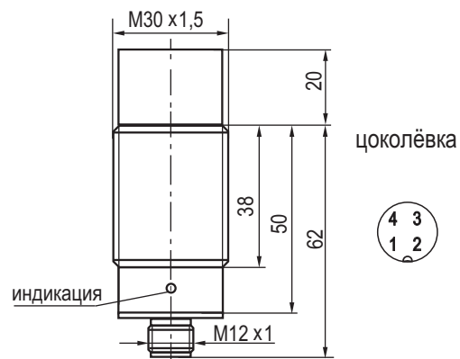
Габаритный чертеж
