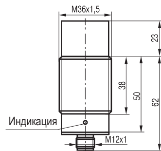
Габаритный чертеж
