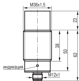
Габаритный чертеж
