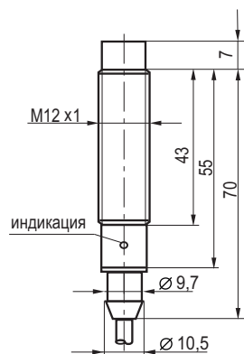
Габаритный чертеж
