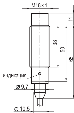
Габаритный чертеж
