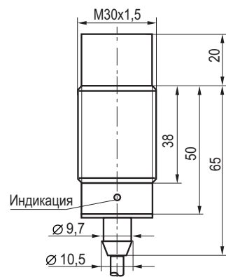
Габаритный чертеж
