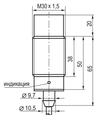
Габаритный чертеж
