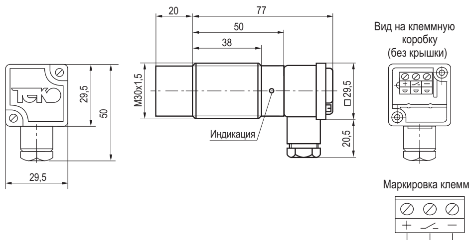
Габаритный чертеж
