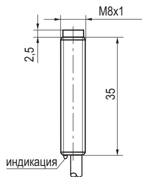
Габаритный чертеж
