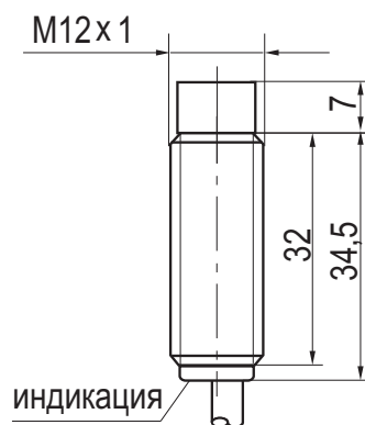
Габаритный чертеж
