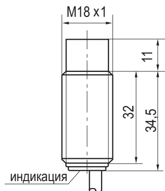
Габаритный чертеж
