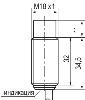
Габаритный чертеж
