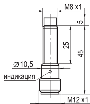
Габаритный чертёж
