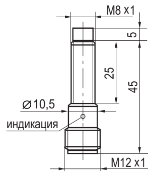
Габаритный чертеж
