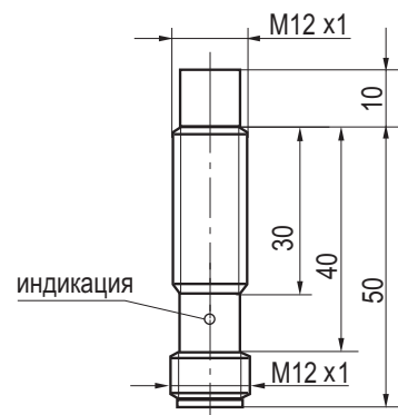
Габаритный чертеж
