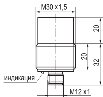
Габаритный чертеж
