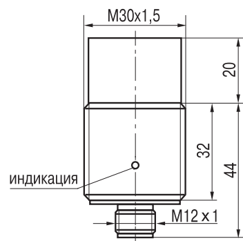
Габаритный чертеж
