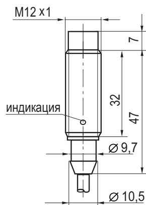
Габаритный чертеж
