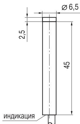
Габаритный чертеж
