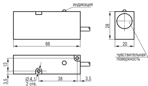
Габаритный чертеж
