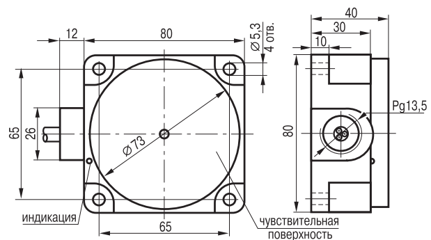
Габаритный чертеж
