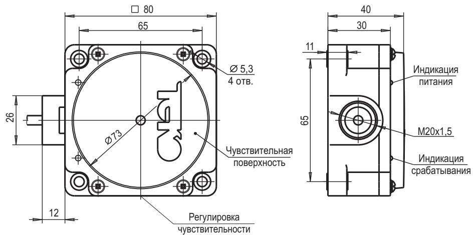
Габаритный чертеж
