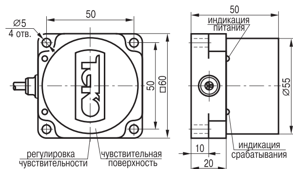
Габаритный чертеж
