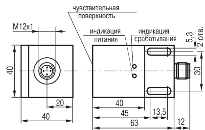
Габаритный чертеж
