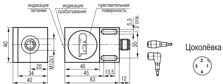
Габаритный чертеж
