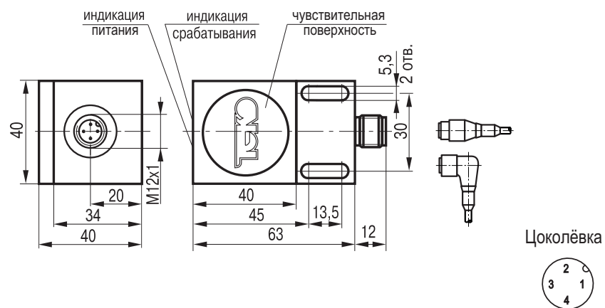
Габаритный чертеж
