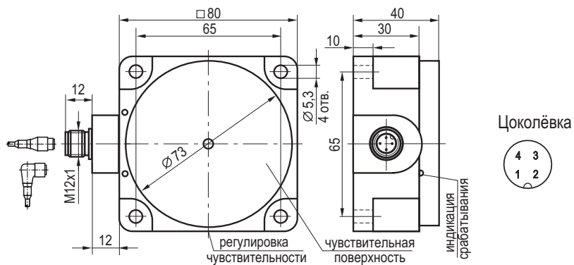
Габаритный чертеж
