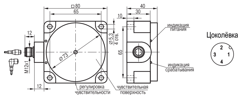
Габаритный чертеж
