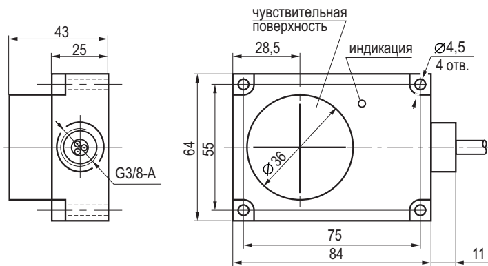
Габаритный чертеж
