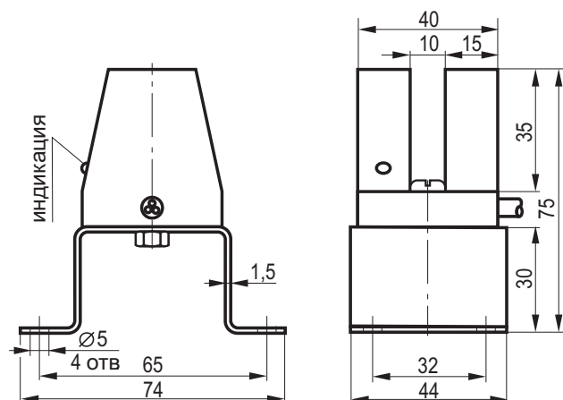
Габаритный чертеж
