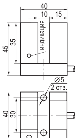
Габаритный чертеж
