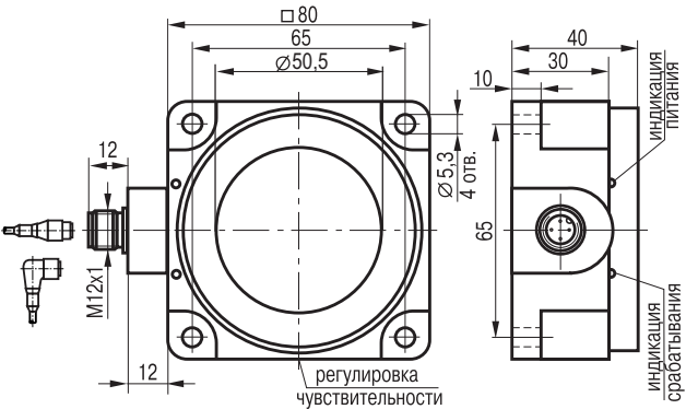
Габаритный чертеж
