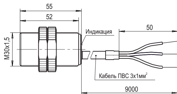
Габаритный чертеж
