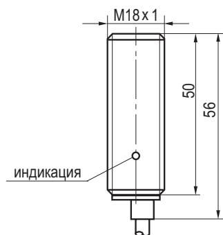
Габаритный чертеж.
